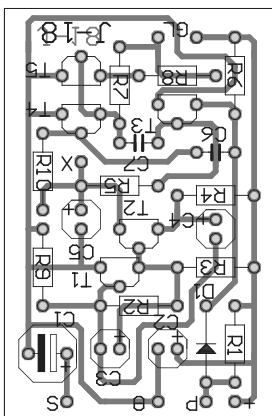
Schemat montażowy
