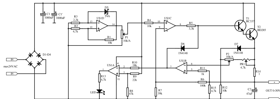
Schemat ideowy
