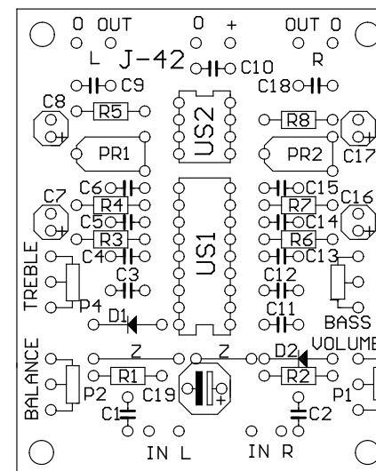
Schemat montażowy
