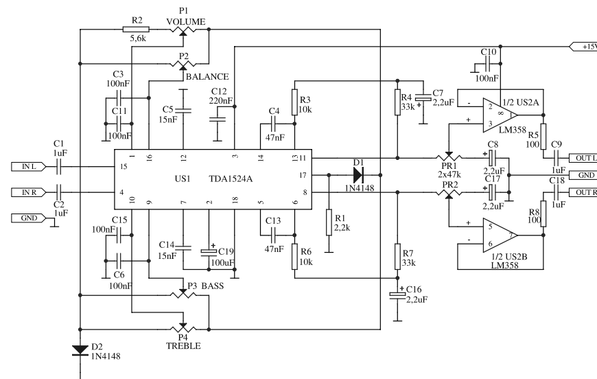
Schemat ideowy
