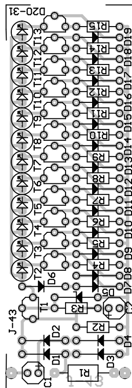
Schemat montażowy
